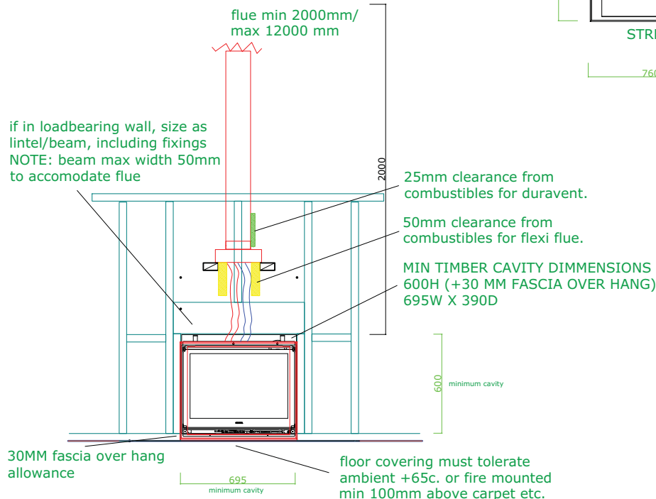
2 ELEVATION Scale: 1:20 @ A3
