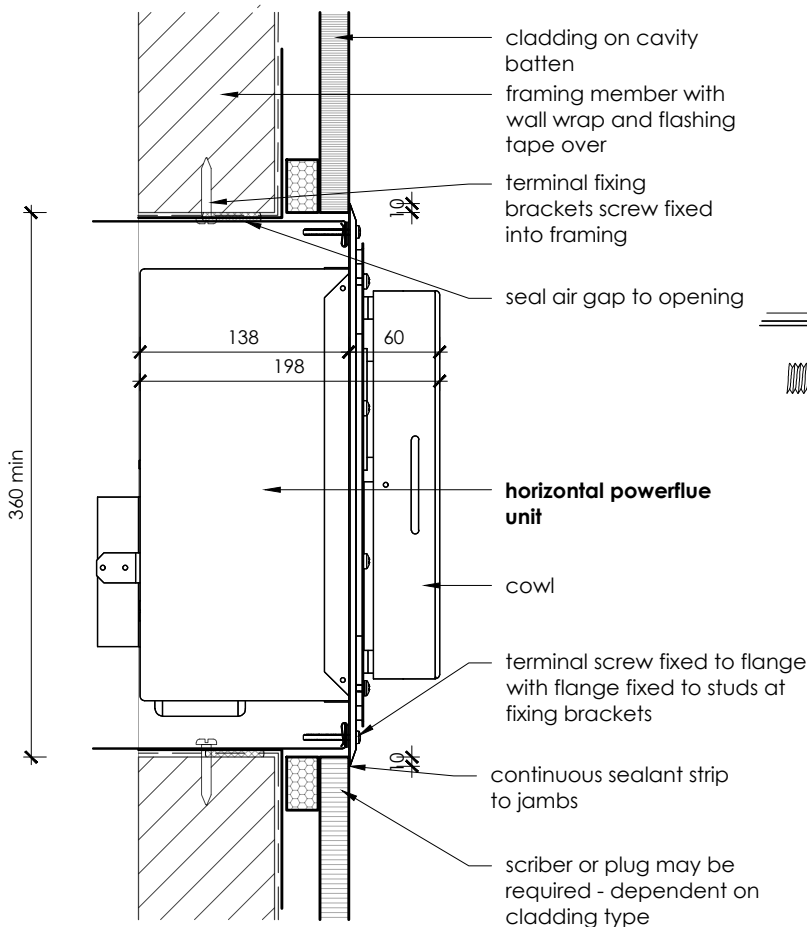
Jamb scale 1:5
