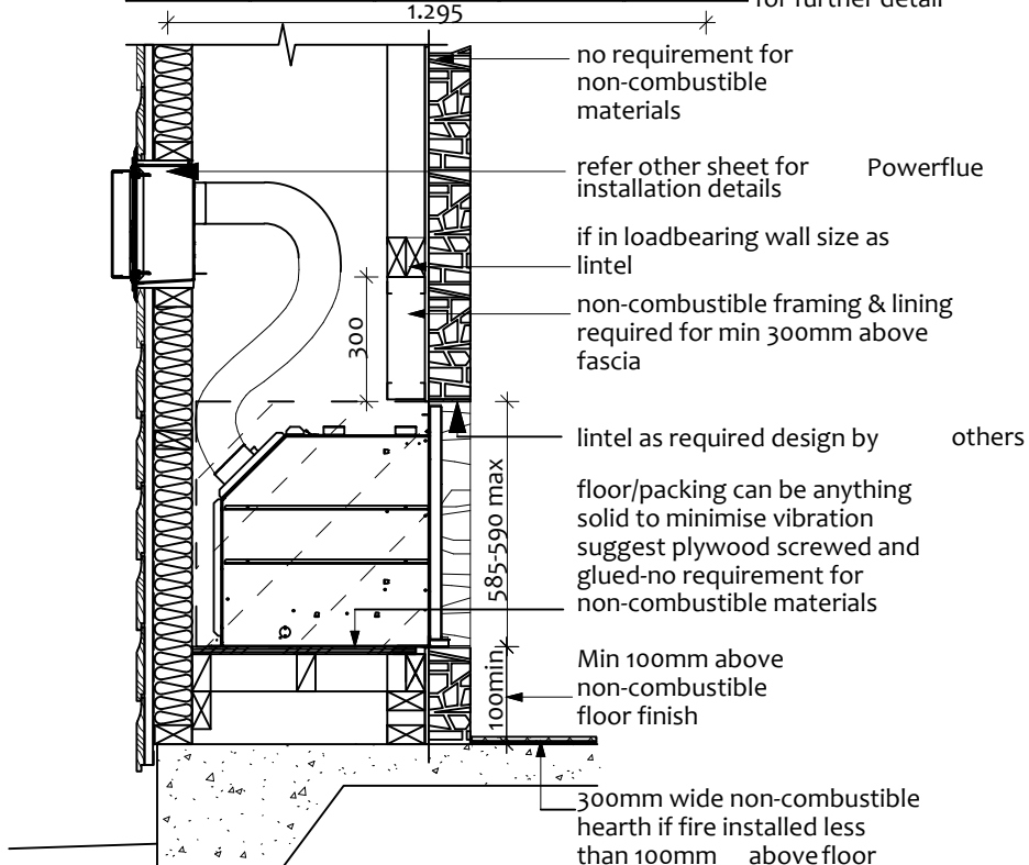
2 CROSS SECTION Scale: 1:20
