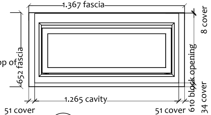
4 FASCIA DIMENSIONS Scale: 1:20
