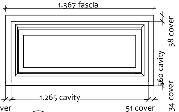
FASCIA DIMENSIONS Scale: 1:20
