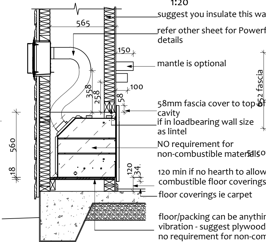
2 CROSS SECTION Scale: 1:20
