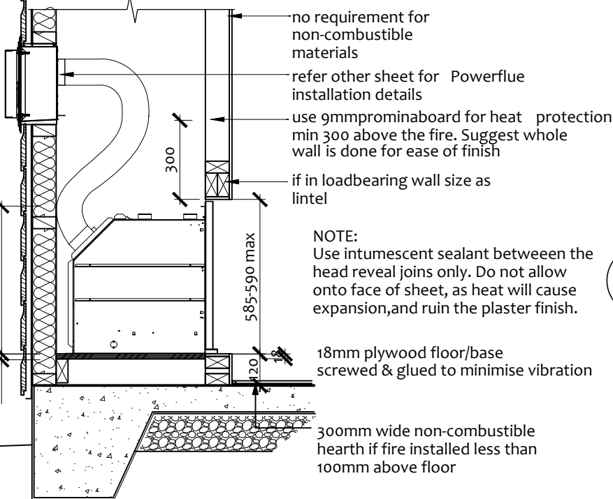
2 CROSS SECTION Scale: 1:20
