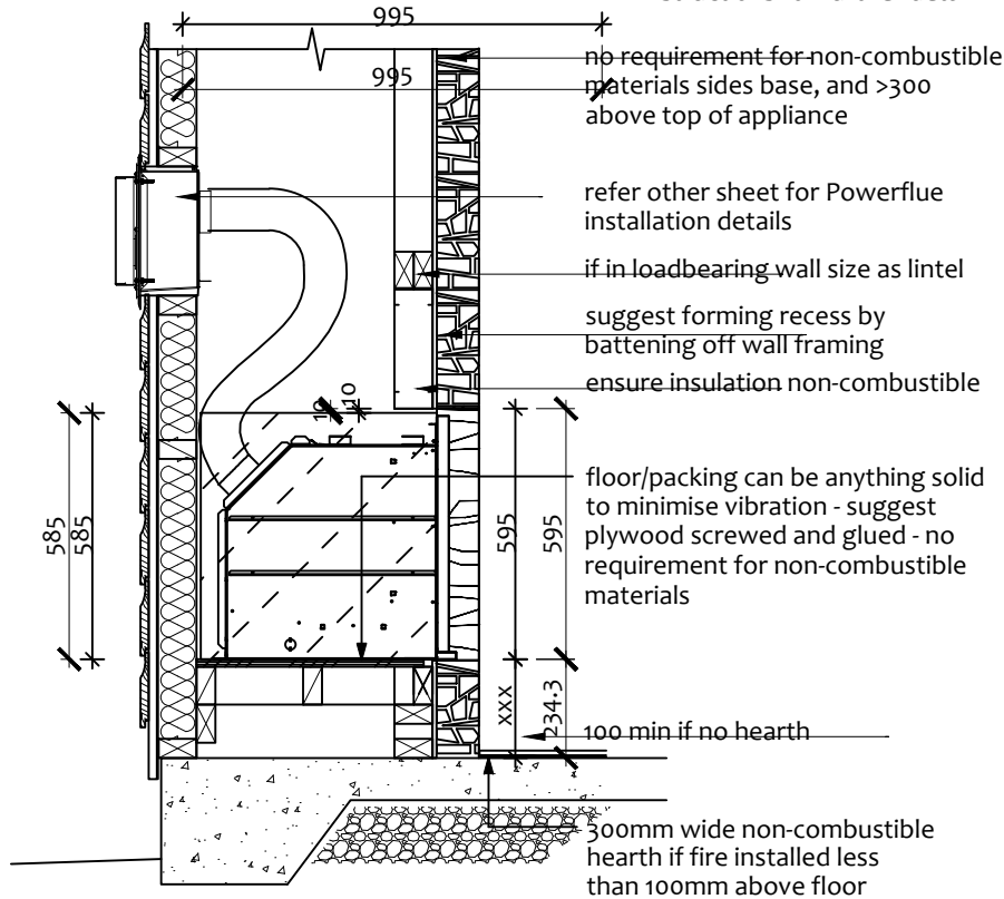
2 CROSS SECTION Scale: 1:20
