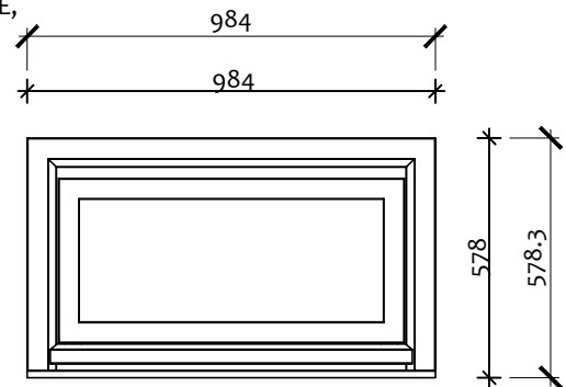
4 FASCIA DIMENSIONS Scale: 1:20
