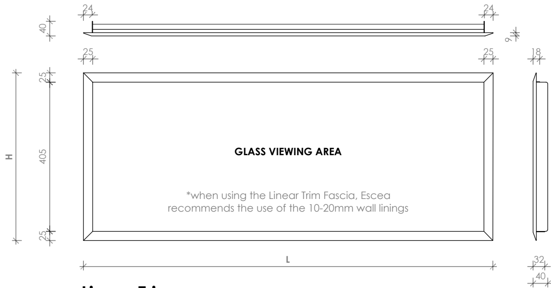
Linear Trim scale 1:10
