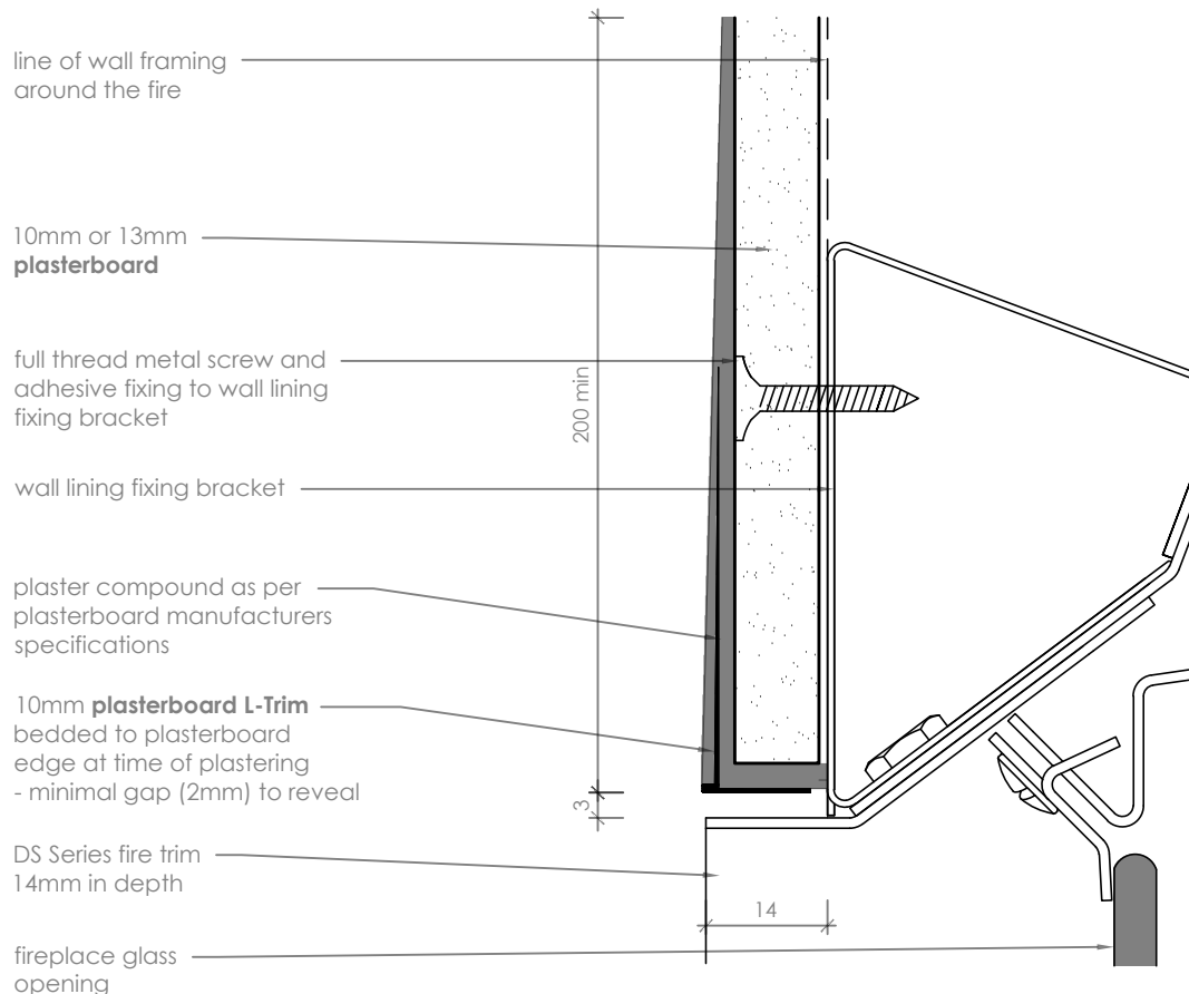
L-Trim Detail
