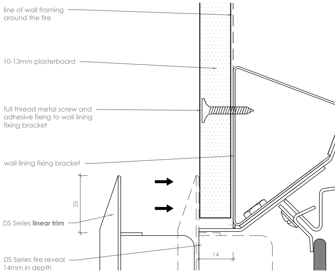
Linear trim
