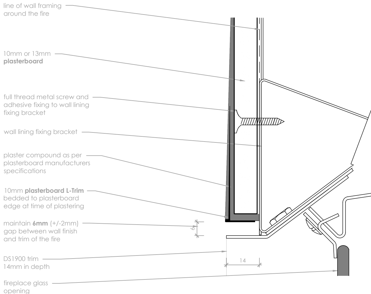
L-Trim Detail
