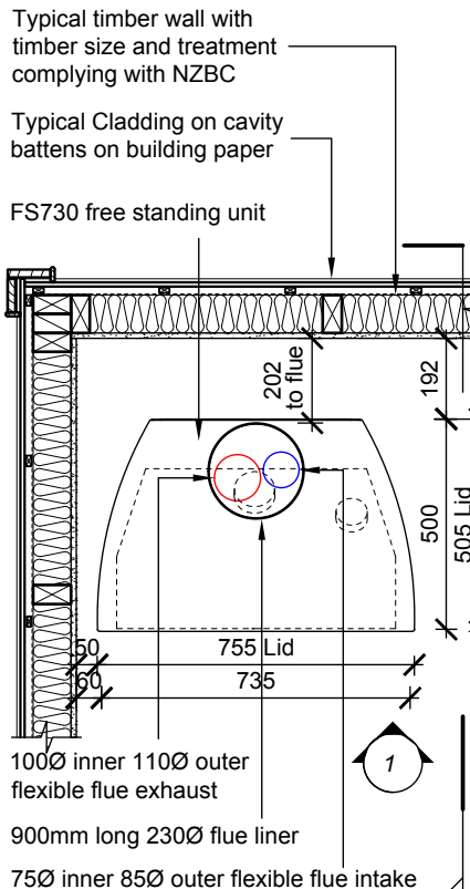
A PLAN Scale: 1:20
