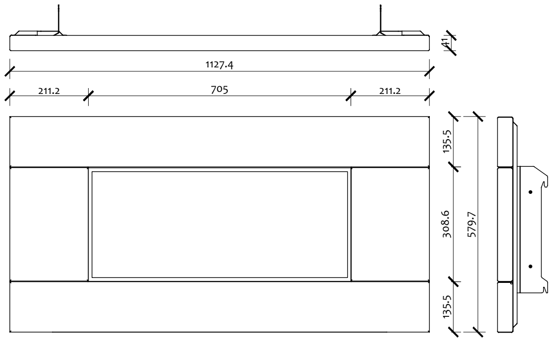
○ ST900 FERRO/SLAB FASCIA Scale: 1:10
